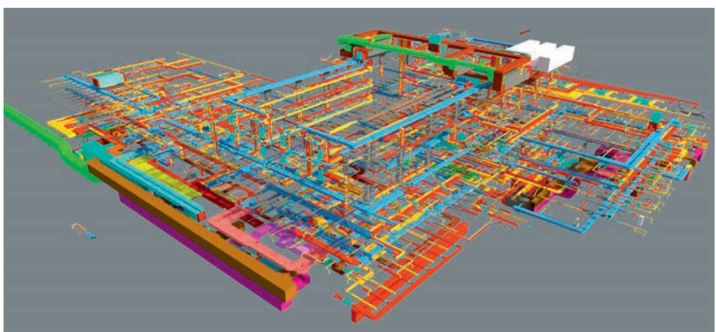
Rohbau- und Haustechnikmodell des Neubaus Spital Limmattal.
